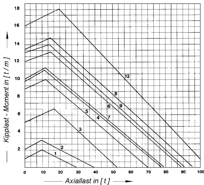
Belastungskurve [ 5 ]
